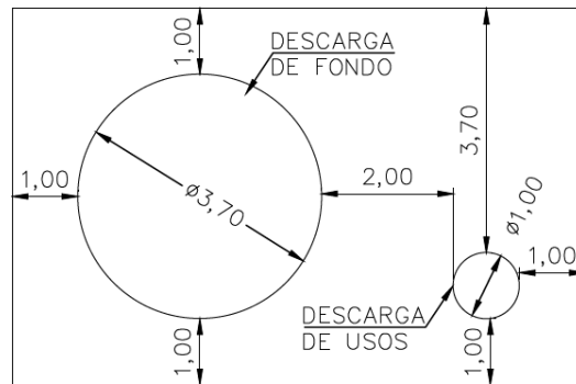
Figura 4. Esquema de descarga de fondo y descarga de usos
