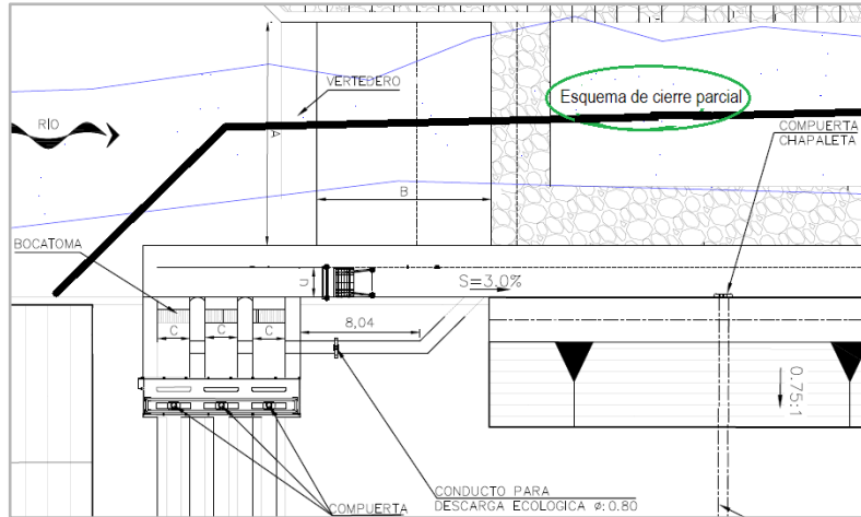
Figura 5. Esquema de cierre parcial
